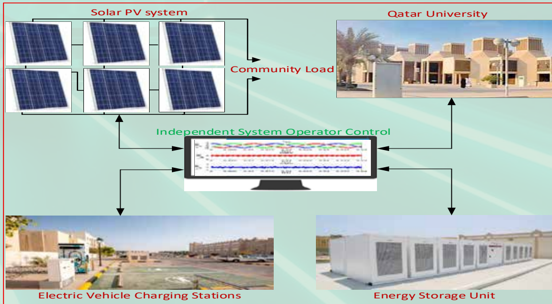
الشكل (1): صور توضيحية لشحن المركبات الكهربائية المدمج مع أنظمة الطاقة الكهروضوئية والتحكم في وحدات تخزين الطاقة من خلال مُشغّل مستقل للنظام.
