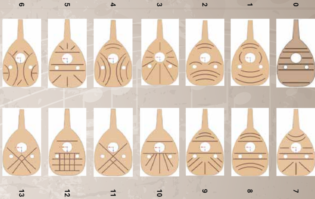
الشكل (1): أربعة عشر نموذجاً مختلفاً من أنظمة تدعيم القُود.
